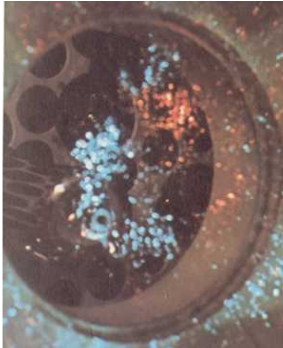
Núcleo de un reactor nuclear. Las manchas oscuras son los huecos en los que están colocadas las barras de uranio.
