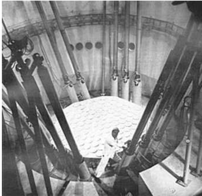
Barras de control en un reactor nuclear de piscina,
