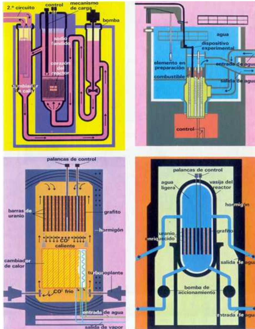
Arriba: a la izquierda, reactor refrigerado por sodio fundido; a la derecha, reactor experimental del tipo piscina. Abajo: a la izquierda, reactor refrigerado por gas; a la derecha, reactor refrigerado y moderado por agua.
