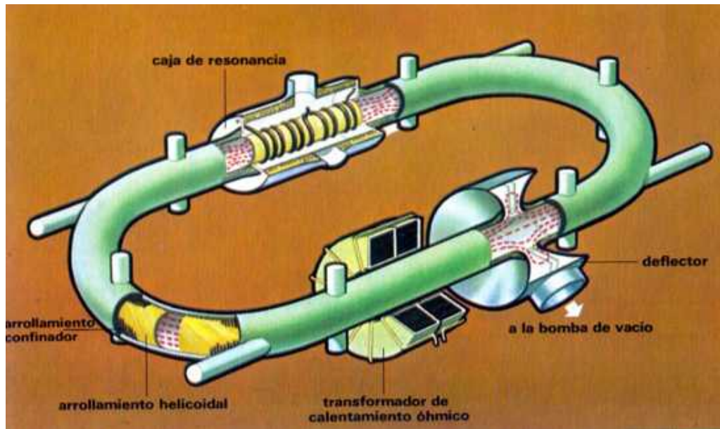
Esquema de un Stellarator en forma de pista de carreras
