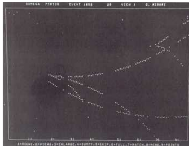
Reconstrucción, obtenida mediante un ordenador, de las sucesivas posiciones de partículas subatómicas en interacción.
