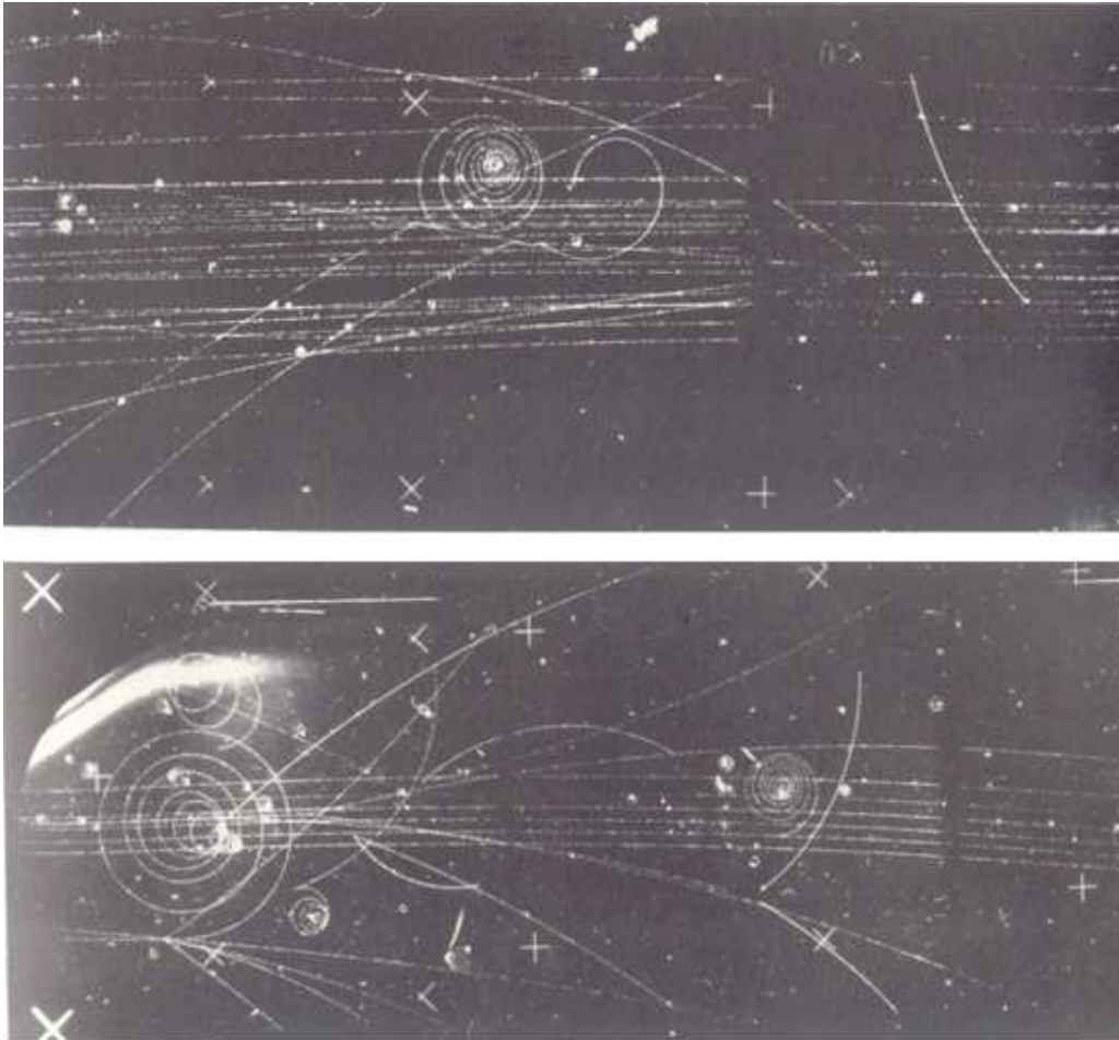
Trazas de partículas elementales obtenidas en una cámara de burbujas sometidas a un fuerte campo magnético.
