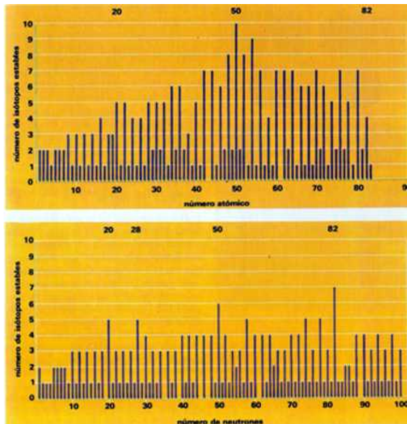
Número de isótopos estables de los distintos elementos en función del número de protones y de neutrones que contiene el núcleo.
