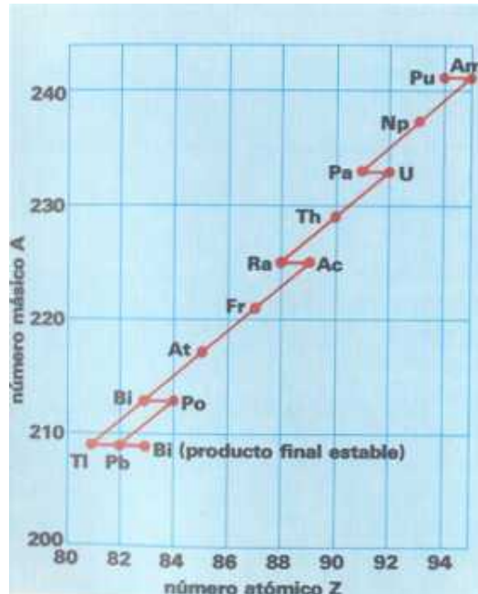
Elementos de la familia radiactiva del neptunio.
