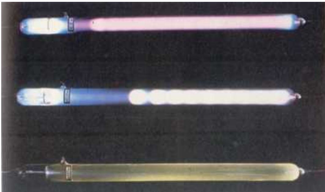
Tubos en los que se produce una descarga luminiscente. Los gases excitados emiten radiación al saltar los electrones atómicos a niveles de menor energía.
