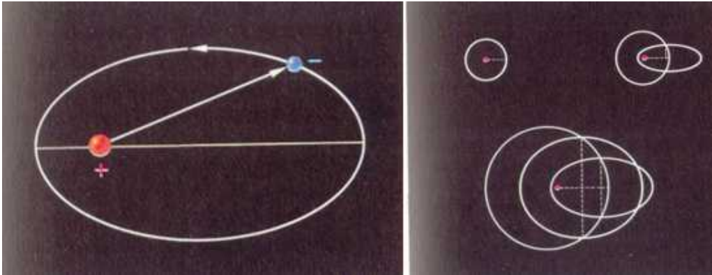
Órbitas elípticas de los electrones alrededor del núcleo atómico.
