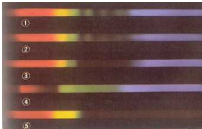
Espectros con bandas de absorción producidas por disoluciones de permanganato potásico a distintas concentraciones (1, 2 y 3), y por filtros de cristal coloreado (4 y 5).
