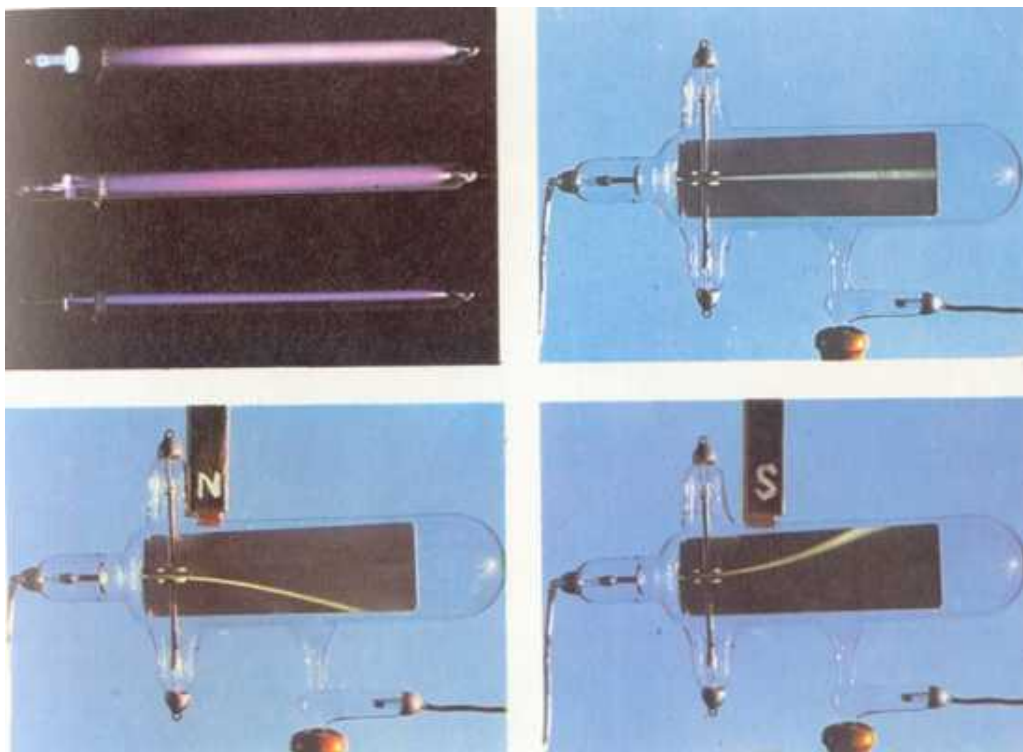
Arriba, descarga luminiscente en tubos con mercurio a diferentes presiones y trayectoria rectilínea de los rayos catódicos. Abajo, desviación de los rayos catódicos por efecto de un campo magnético (imán).
