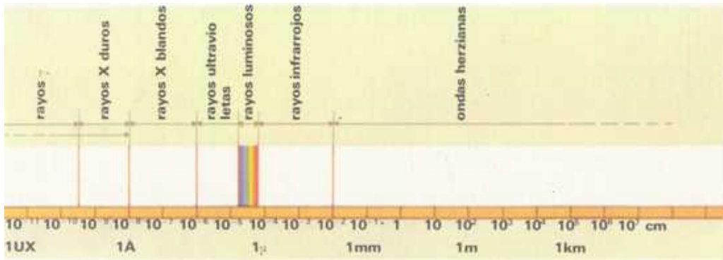
Espectro electromagnético. Distribución de las radiaciones en función de la longitud de onda.
