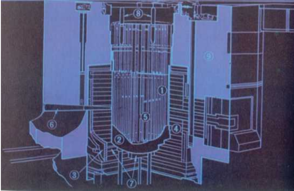
Interior del reactor nuclear JJR-3. 1, barras de combustible; 2, paredes del núcleo; 3, aislador térmico; 4, reflector de grafito; 5 y 6, huecos para la práctica de experimentos; 7, isótopos; 8, barras de control; 9, pantalla protectora.
