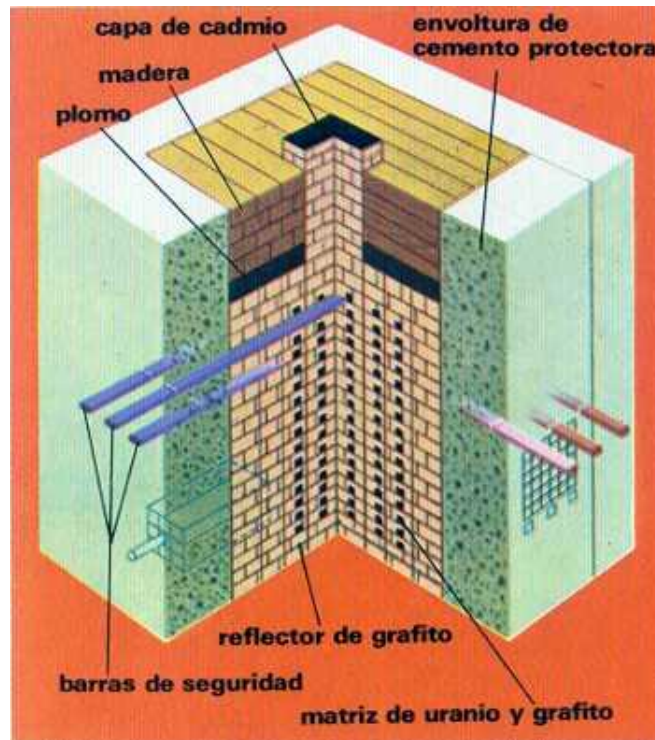
Esquema del núcleo de un reactor de uranio natural y grafito.
