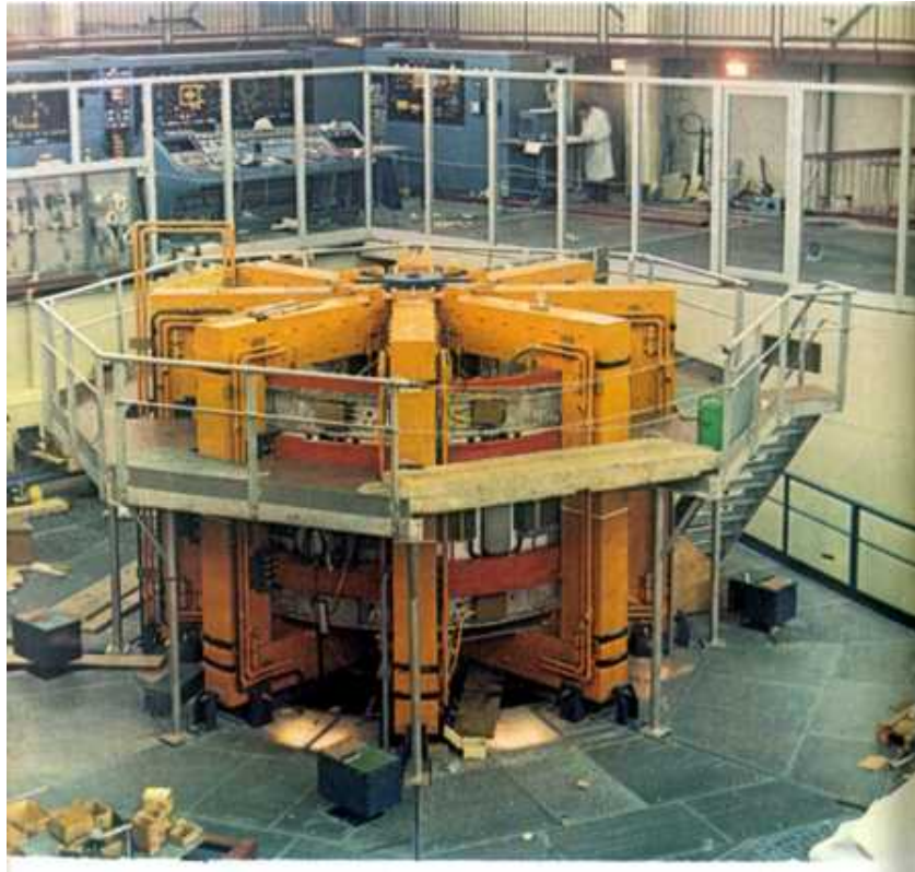
Instalaciones del reactor Tokomat (URSS).
