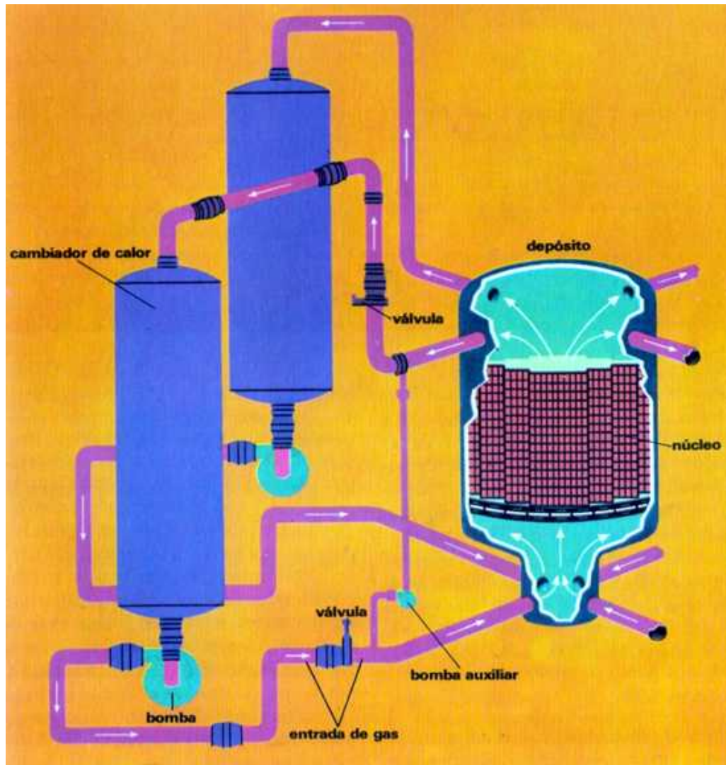
Esquema del reactor nuclear de Calder Hall (Escocia) de uranio natural moderado con grafito.
