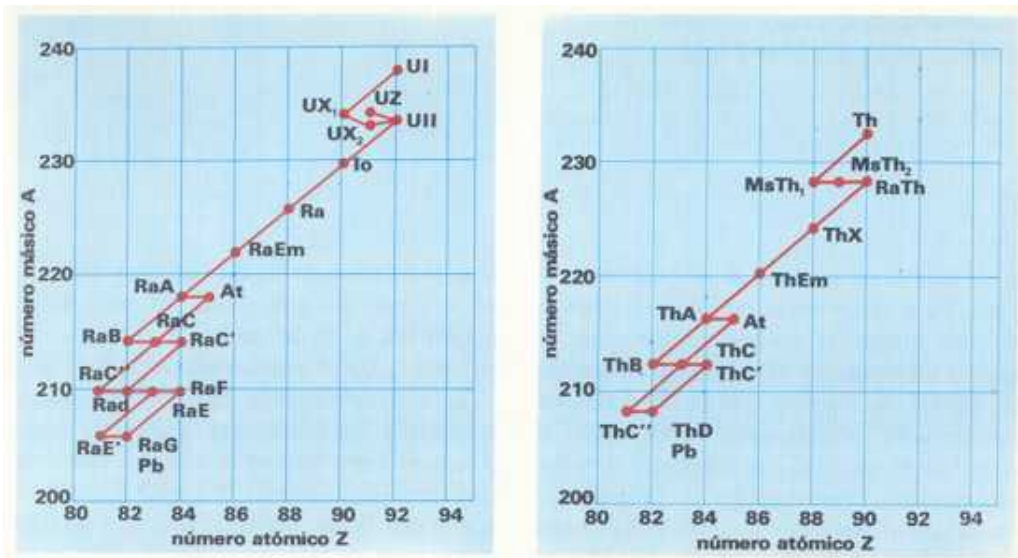
Familias radiactivas del uranio (izquierda), del torio (derecha) y del actinio (abajo). Las líneas inclinadas corresponden a transmutaciones producidas por emisión de una partícula \alpha , y las horizontales, a transmutaciones producidas por emisión de una partícula \beta^- .
