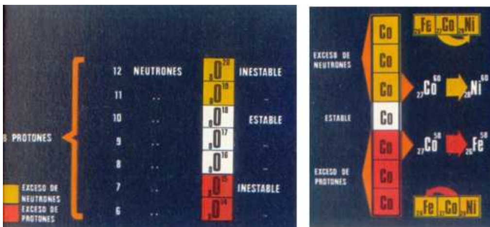
Los núcleos con un exceso de protones o de neutrones son inestables. Isótopos estables e inestables del oxígeno (izquierda) y del cobalto (derecha).
