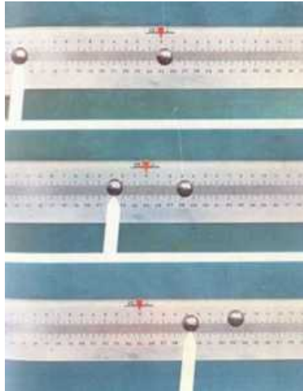
La repulsión entre cargas de distinto signo varía con su distancia.
