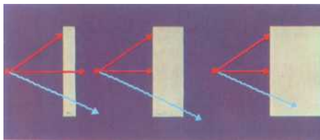
Distinto poder de penetración de los rayos \alpha , \beta y \gamma en la materia.
