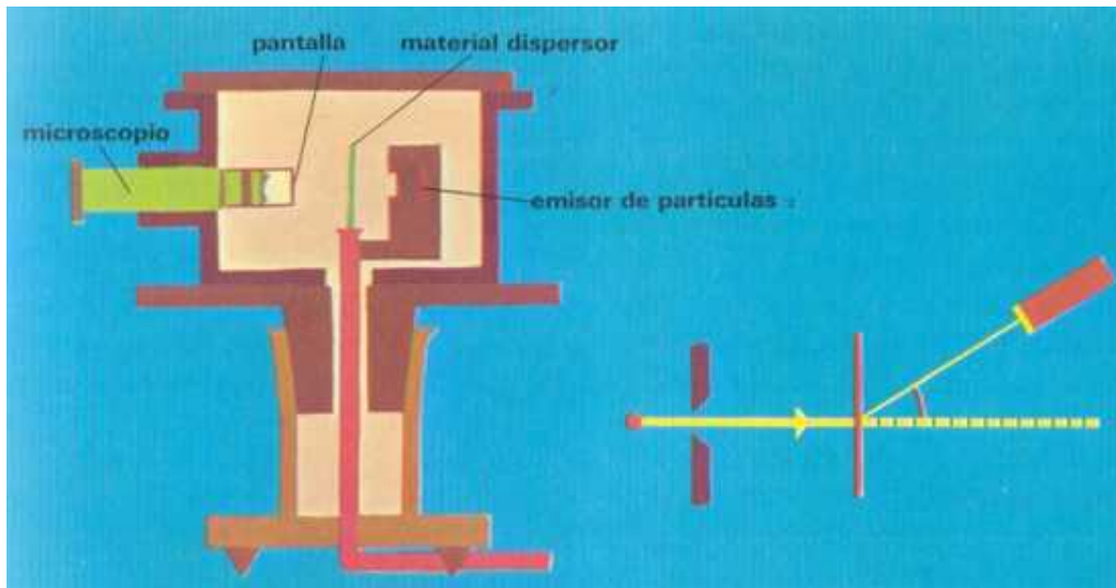
Esquemas del dispositivo experimental utilizado por Geiger y Marsden. El giro del microscopio (a la derecha) permite detectar las partículas alfa dispersadas en diversas direcciones.
