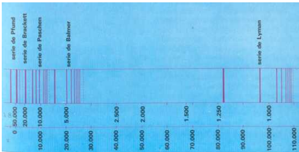
Posición relativa de las series espectrales del átomo de hidrógeno.
