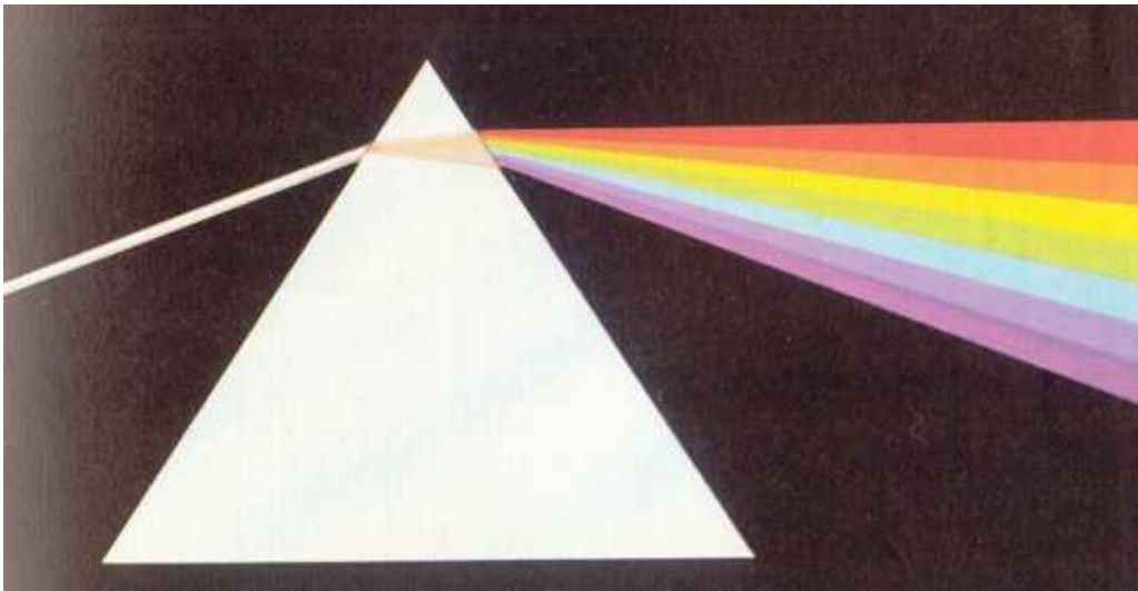
Descomposición de la luz blanca en los siete colores del espectro por medio de un prisma.
