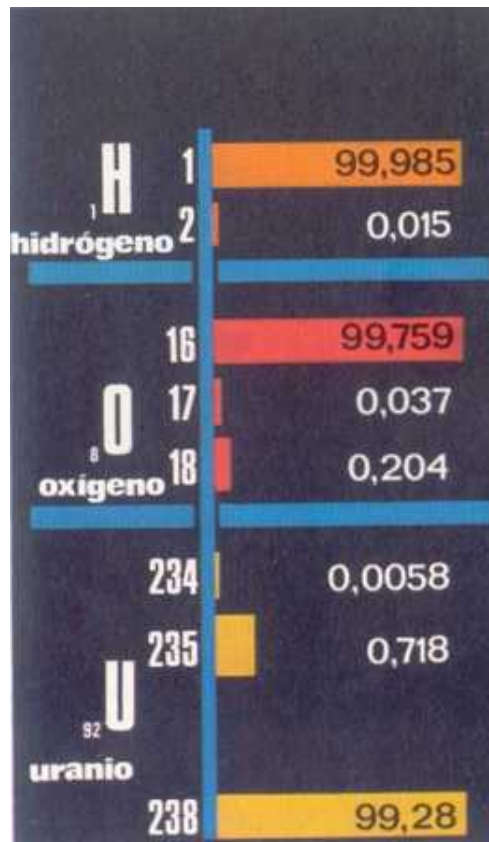
Isótopos de algunos elementos y su abundancia relativa en tantos por ciento.
