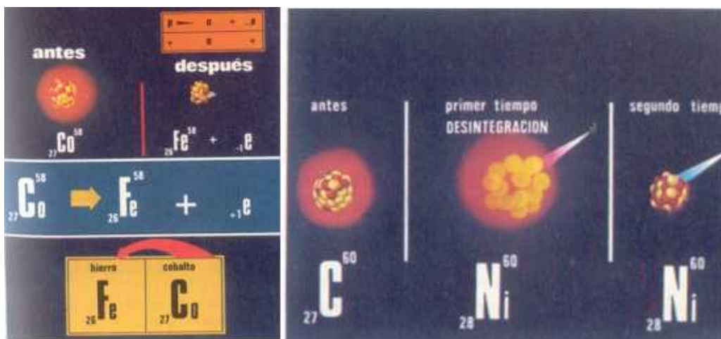
Transmutación radiactiva de una partícula \beta^+ o _{+1}e (izquierda) y por emisión de una partícula \beta^- seguida de la emisión de radiación \gamma (derecha).
