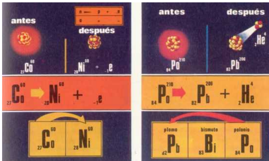
Transmutaciones radiactivas producidas por emisión de una partícula \beta^- o {}_{-1}^0\text{e} (izquierda), de una partícula \alpha o {}_{2}^4\text{He} (derecha)
