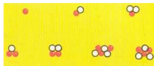
Isótopos del hidrógeno (1 protón), helio (2 protones) y litio (3 protones); los protones aparecen en rojo y los neutrones en blanco.
