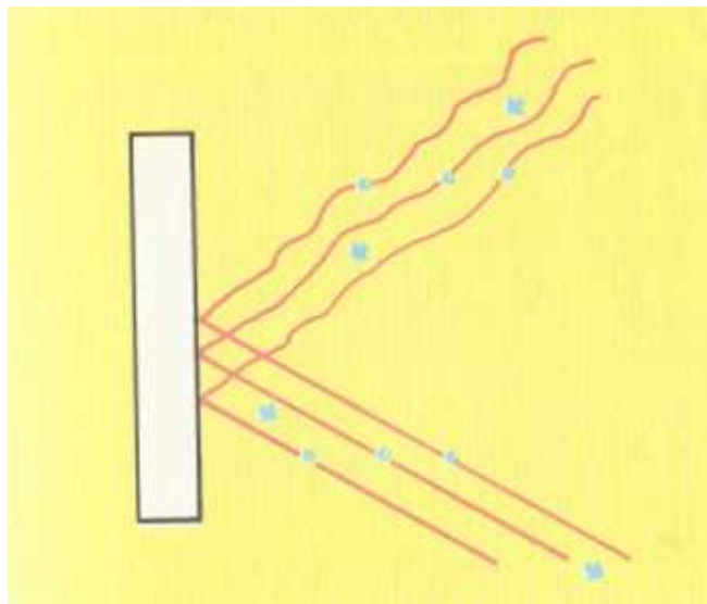
El efecto fotoeléctrico consiste en la emisión de electrones por una sustancia sometida a un bombardeo de fotones.
