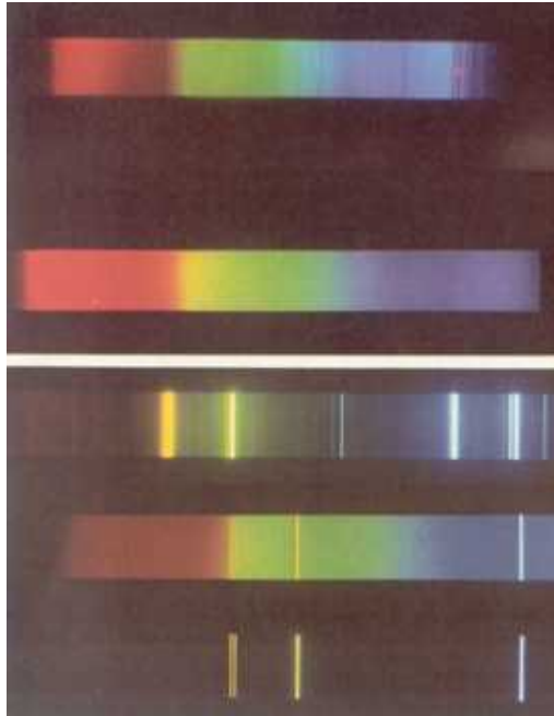
Espectros ópticos. Arriba, espectro de la luz solar en el que aparecen líneas de absorción (líneas de Fraunhofer) y espectro de la luz de una candela; abajo, espectros emitidos por lámparas de mercurio, en diferentes condiciones.
