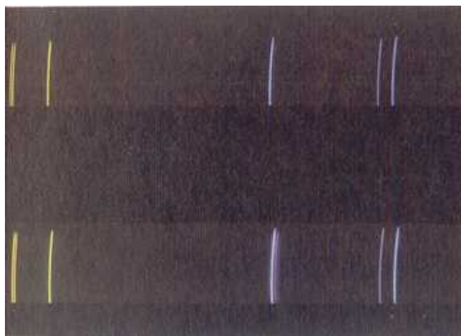
Líneas del espectro de emisión del mercurio.
