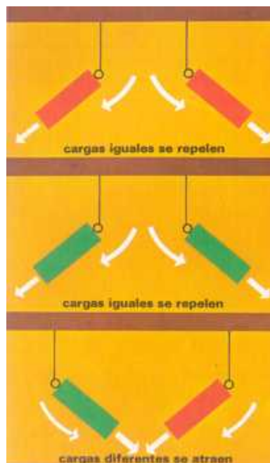
Representación de la acción mutua entre cargas eléctricas.
