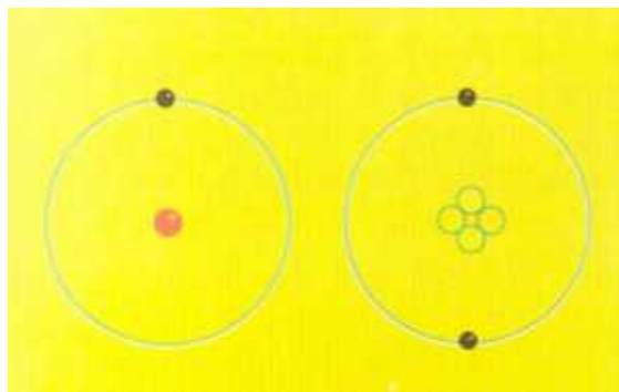
Representación esquemática de los átomos de hidrógeno y del helio.
