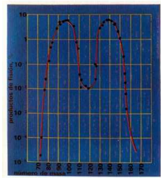
Distribución en tanto por ciento de los productos de la fisión de un núcleo pesado.
