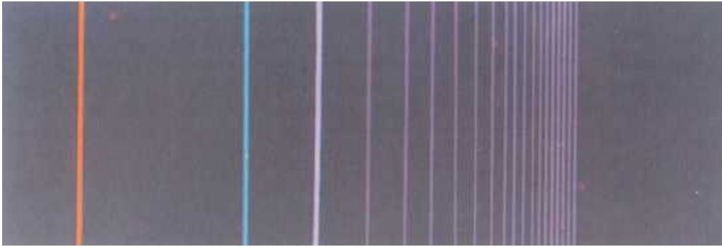
Líneas espectrales de la serie de Balmer del átomo de hidrógeno.
